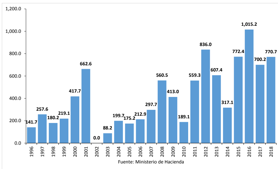
Gráfico No. 9 LETES: Saldos Anuales 1996 -2018 (valor precio) (Millones de US$)
